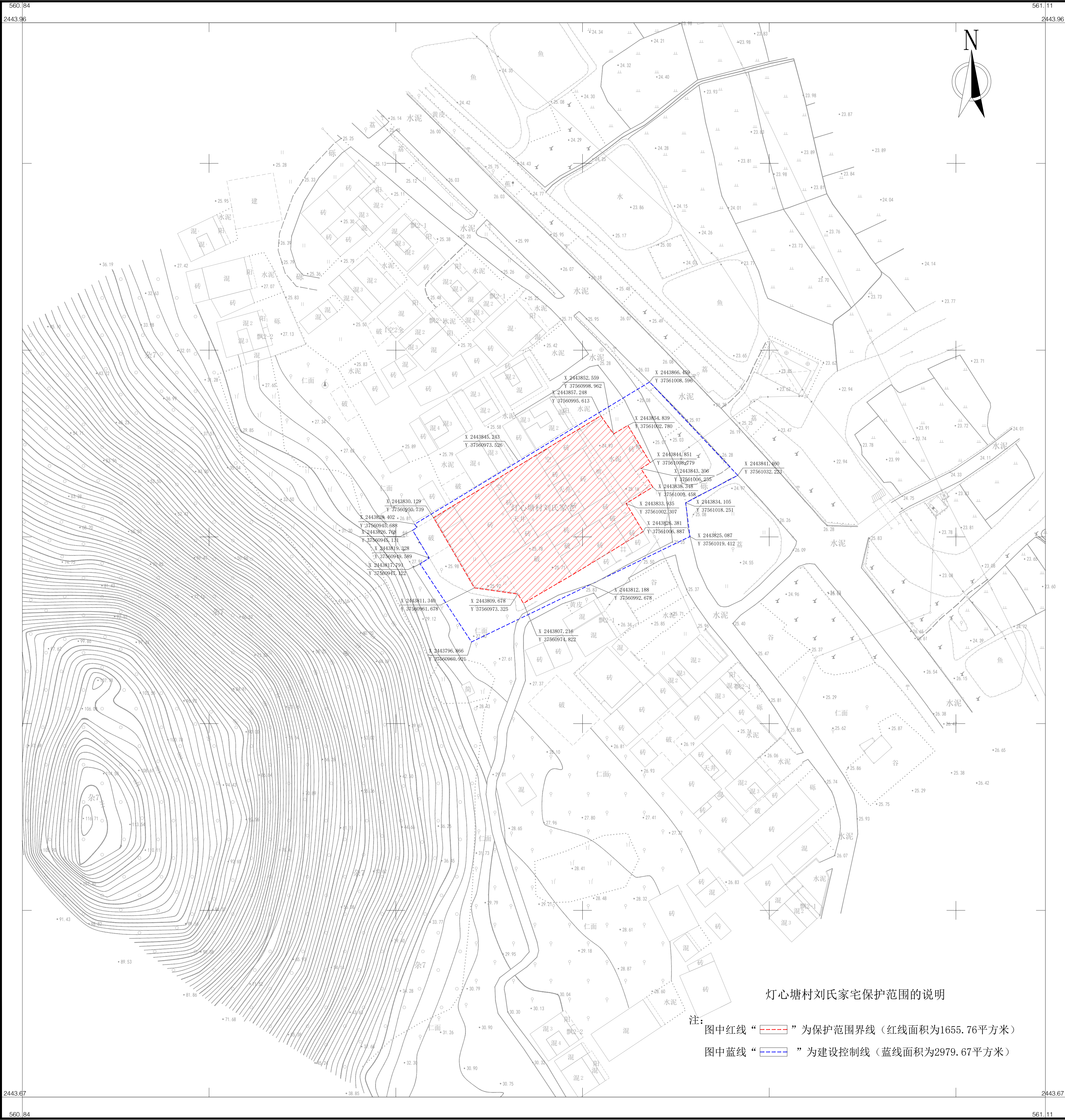
灯心塘村刘氏家宅1：500地形图
