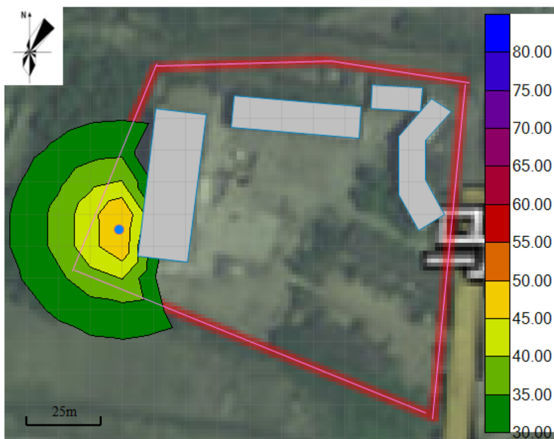
图 7-2 项目噪声预测等声级线图 单位：dB（A）
