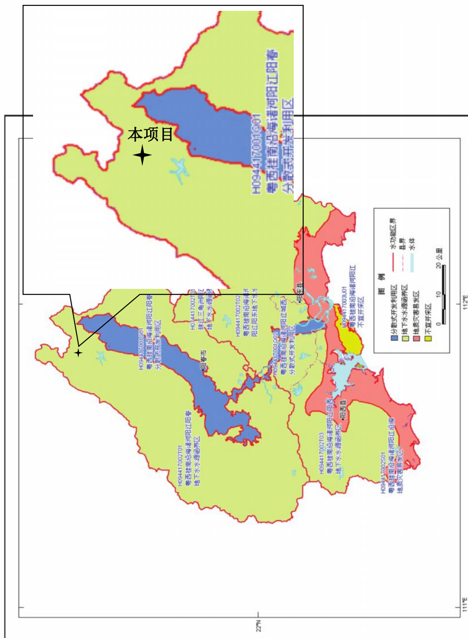
图 16 阳江市浅层地下水功能区划图
