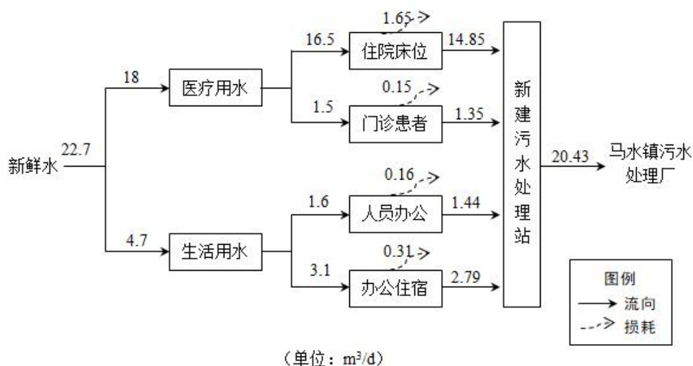
图 1-1 项目水平衡图
