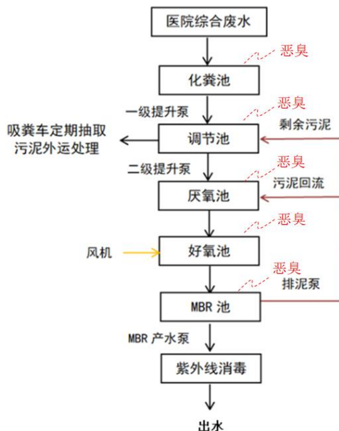
图7-1 污水处理站工艺流程图
