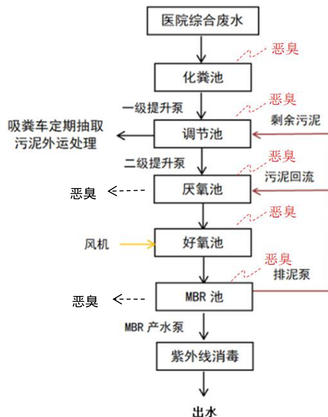
图 5-3 污水处理站工艺流程图
